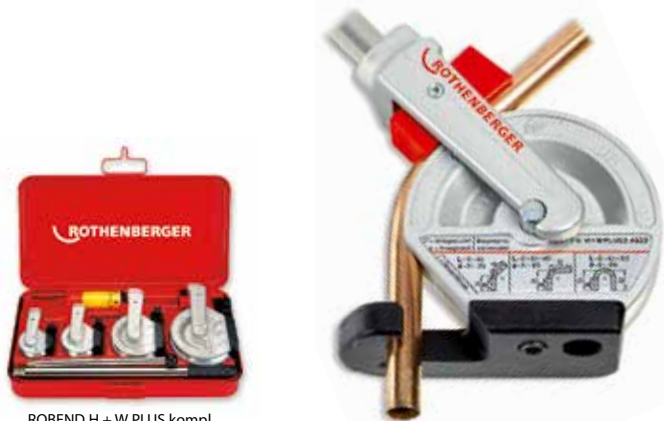
ROBEND H + W PLUS kompl.
